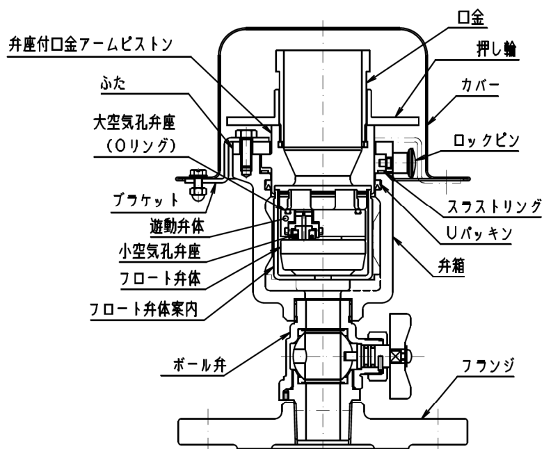
呼び径 25 フランジ付きねじ込み形 町野式口金内蔵
