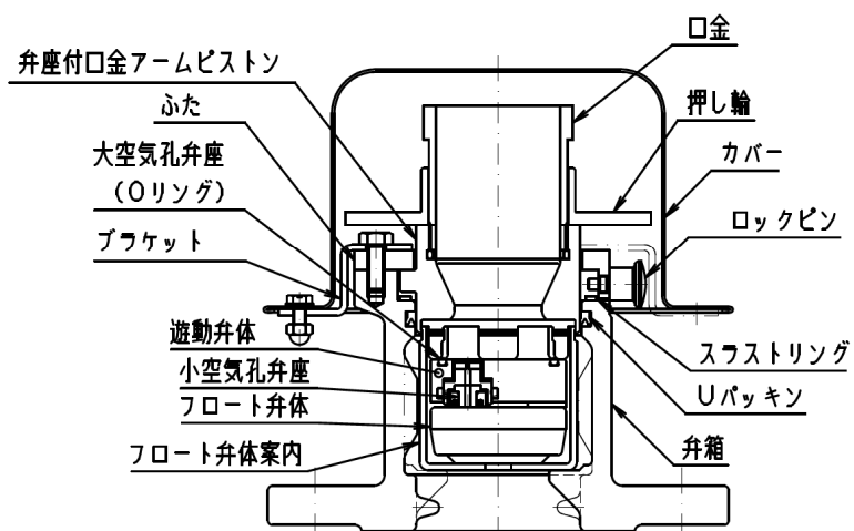
呼び径 25 フランジ一体形 町野式口金内蔵
