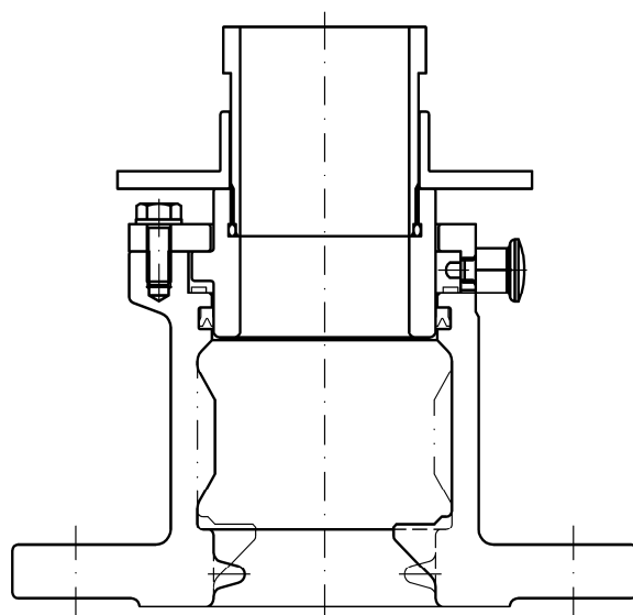
フランジー体形
