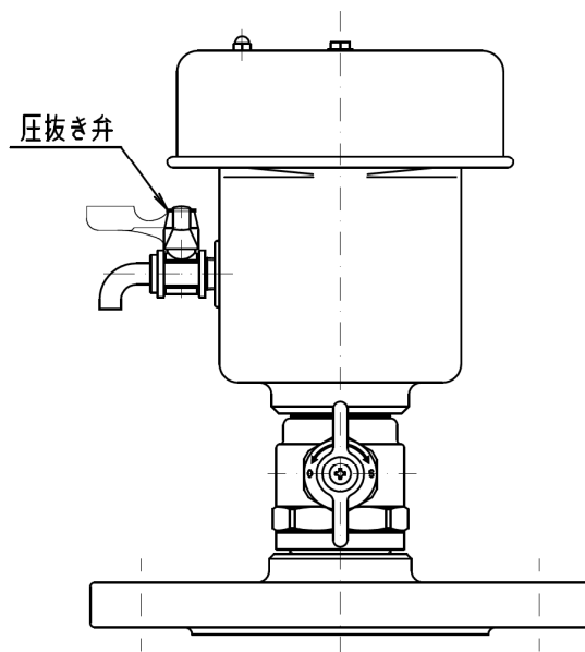
呼び径 25 フランジ付きねじ込み形
