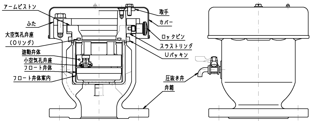
呼び径 75 フランジ形
