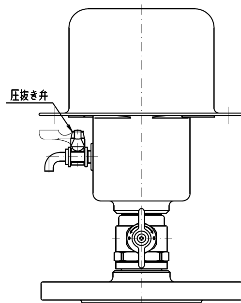
呼び径 25 フランジ付きねじ込み形 町野式口金内蔵
