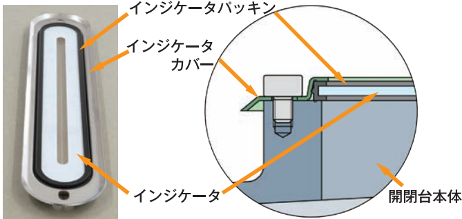
セットした状態(裏側) 弁開度表示(インジケータ)部 構造説明のために色をつけたもので、実際の製品の色とは異なります。
