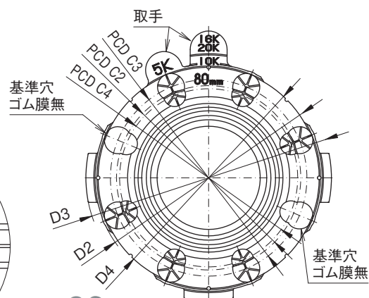
呼び径 80の場合
