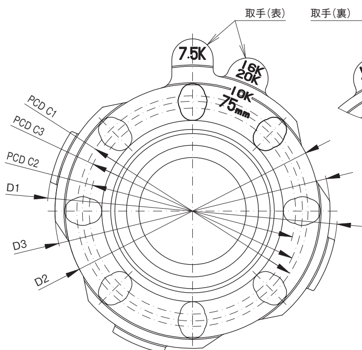
7.5Kフランジの場合
