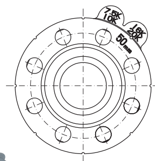
呼び径 50の場合
