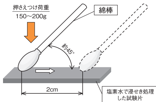
綿棒による測定方法
