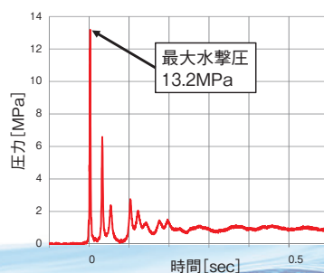
急速空気弁にて発生した水撃圧
